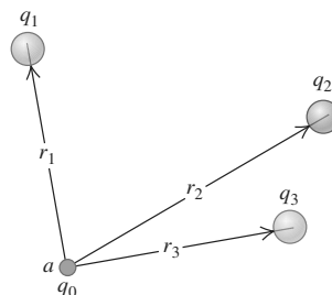
23.8 La energía potencial asociada con la carga q_0 en el punto a depende de las otras cargas q_1, q_2 y q_3 y de sus distancias r_1, r_2 y r_3 desde el punto a .
