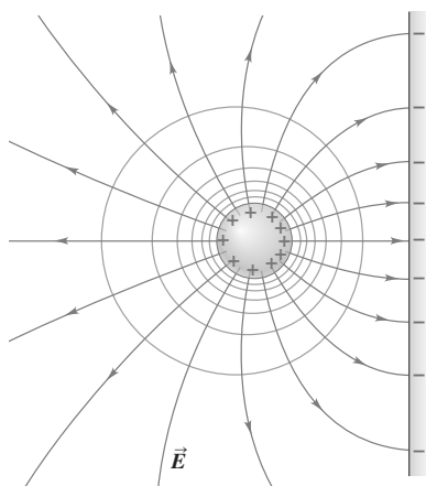
— Secciones transversales de las superficies equipotenciales
